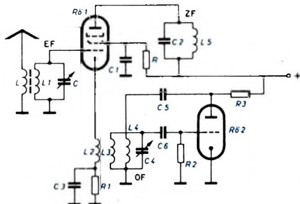
Bild 13. Mischschaltung mit getrenntem Oszillator (Katodenmischung)
