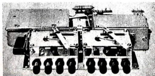
Bild 5. Ansicht der Drucktastenkombination
