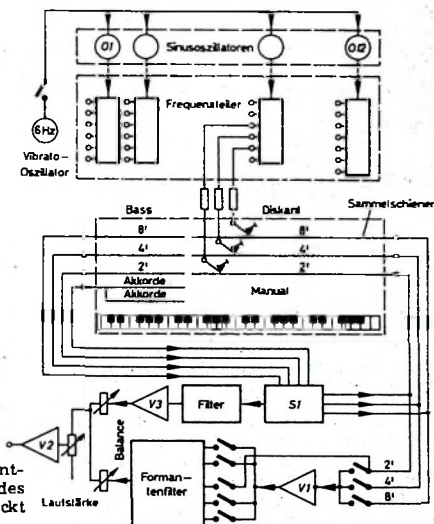
Bild 5. Block-schemata der „Philicorda“
