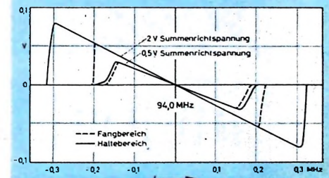
Bild 4. Regelkurven bei 0,5 V und 2 V Summenrichtspannung
