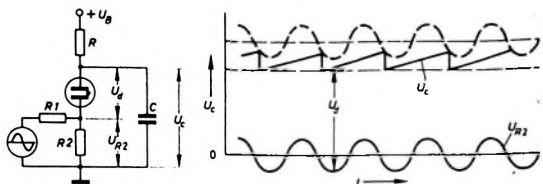
Bild 7. Synchronisierung eines Sägezahn-generators mit einer Sinusspannung
