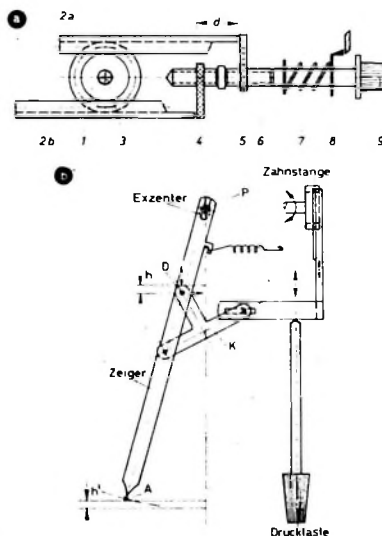
Bild 1. Arbeitsprinzip der Drucktastenabstimmung (a) und des Skalenzeigers (b)
