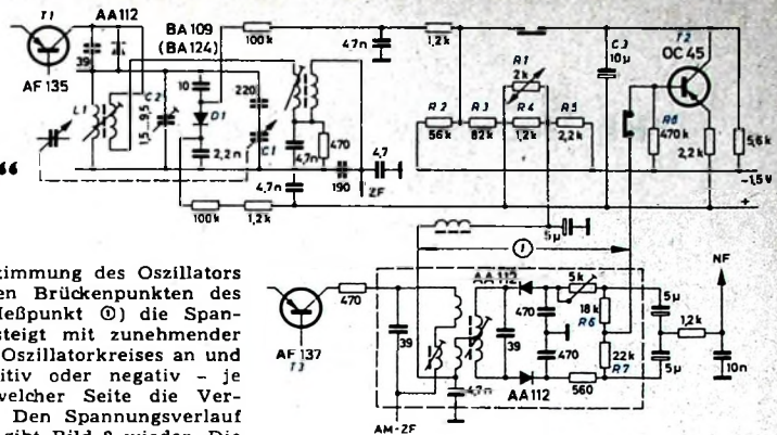
Bild 1. Schaltung der Nachstimmautomatik
