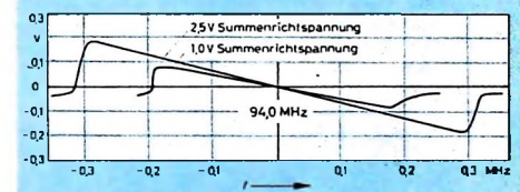
Bild 3. Am Meßpunkt ① bei Verstimmung des Oszillators auftretende Spannungen
