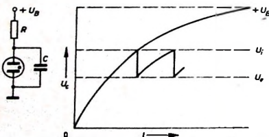
Bild 6. Schaltung (links) und Verlauf der Spannung U_c eines frei laufenden Sägezahn-generators
