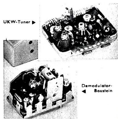
Bild 7. Der entscheidende Baustein für die hohe FM-Empfindlichkeit des „Trans-Amerika-L“ ist der abgeschirmte UKW-Tuner; der ebenfalls abgeschirmte Demodulator-Baustein enthält außer Radiodetektor und AM-Demodulator auch die letzte ZF-Stufe
