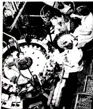
In den Anfangsjahren der Röhrenfertigung wurden die Röhren noch einzeln gepumpt (links); heute sind dafür Pump- und Gatter-Automaten eingesetzt
