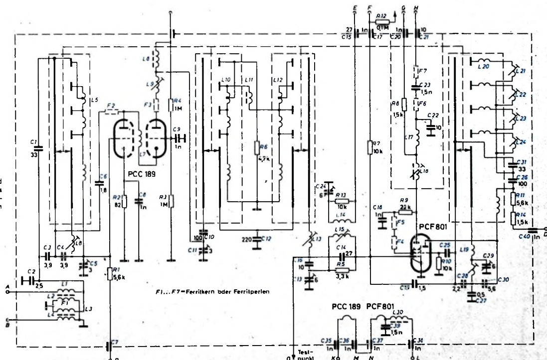
Bild 2. Schaltbild des VHF-Teiles der Kanalwähler-Kombination
