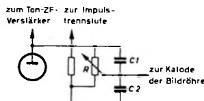
Bild 6. Prinzip der videofrequenten Kontrastregelung
