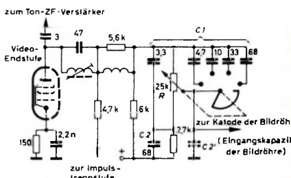
Bild 6. Prinzip der videofrequenten Kontrastregelung
