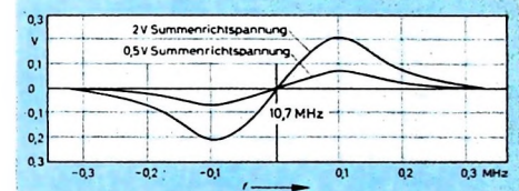
Bild 2. Spannungsverlauf am Meßpunkt ①
