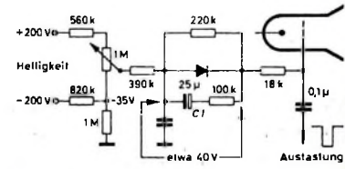
Bild 8. Schaltung der Leuchtfleckunterdrückung
