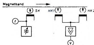
Bild 1 Prinzipschema zur Ermittlung der Bandgeschwindigkeit aus Aufzeichnungsfrequenz und Messung der Wellenlänge mit Hilfe von zwei in ihrem Abstand veränderbaren Hörköpfen HK 1 und HK 2
