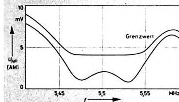
Bild 4. AM-Unterdrückung des Ton-ZF-Verstärkers
