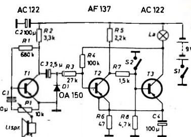
Schaltung des Anzeigegerätes
